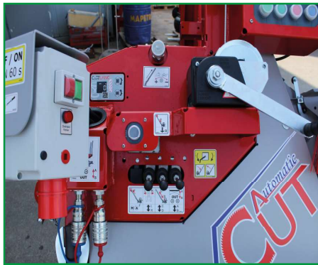
Geschwindigkeitsverstellung des Förderbands
